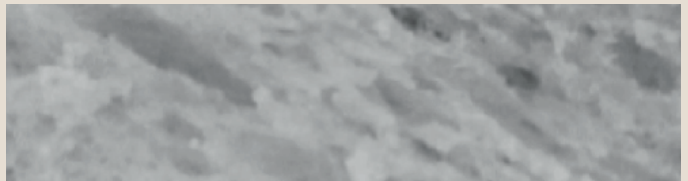
kuchenartige Porung
