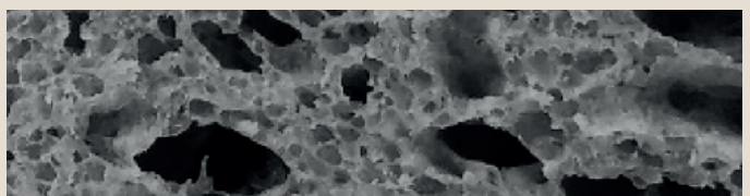
ungleichmäßige Porung
