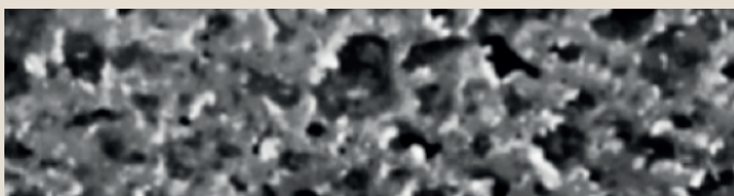
kompakte Porung
